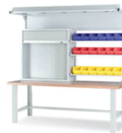
Werkbankaufbau 2000 Modell 4 H × B (mm): 1270 × 2000 2 × Aufbaustütze H = 1270 mm, 1 × Querverbinder 1940 mm, 1 × Zwischenstütze 960mm, 1 × Perfolochwand 1940 × 300 mm, 1 × Rolladenschrank mit Perfolochblech 955 × 955 × 230 mm, 3 × Fachboden 975 × 235 mm Art.-Nr. 033488 886,00 € 2 × Tragarme, Beleuchtung mit 4 LED-Spots und 3 m Anschlusskabel mit Stecker Art.-Nr. 033489 1220,00 €
